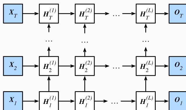
图6.11 深度循环神经网络的架构
