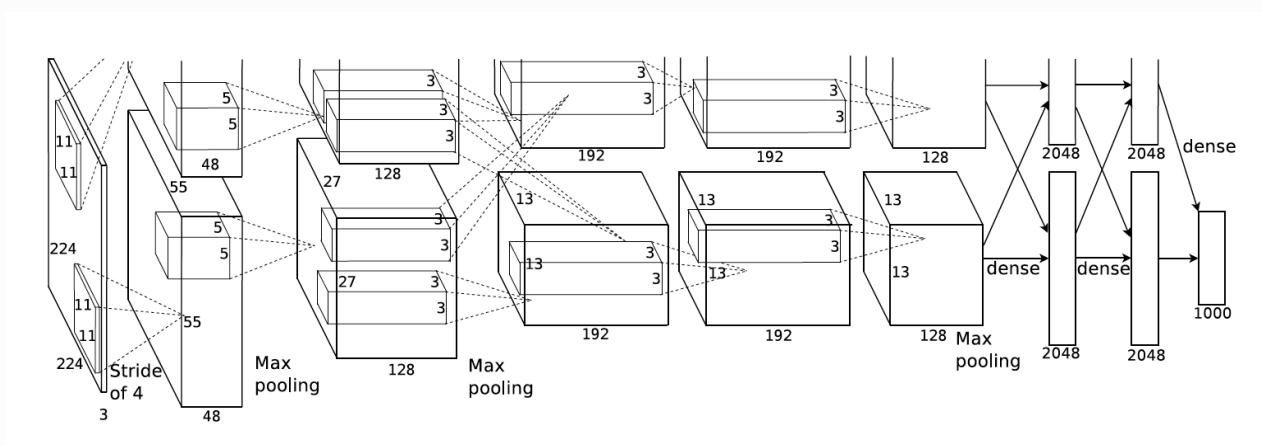
AlexNet网络结构
