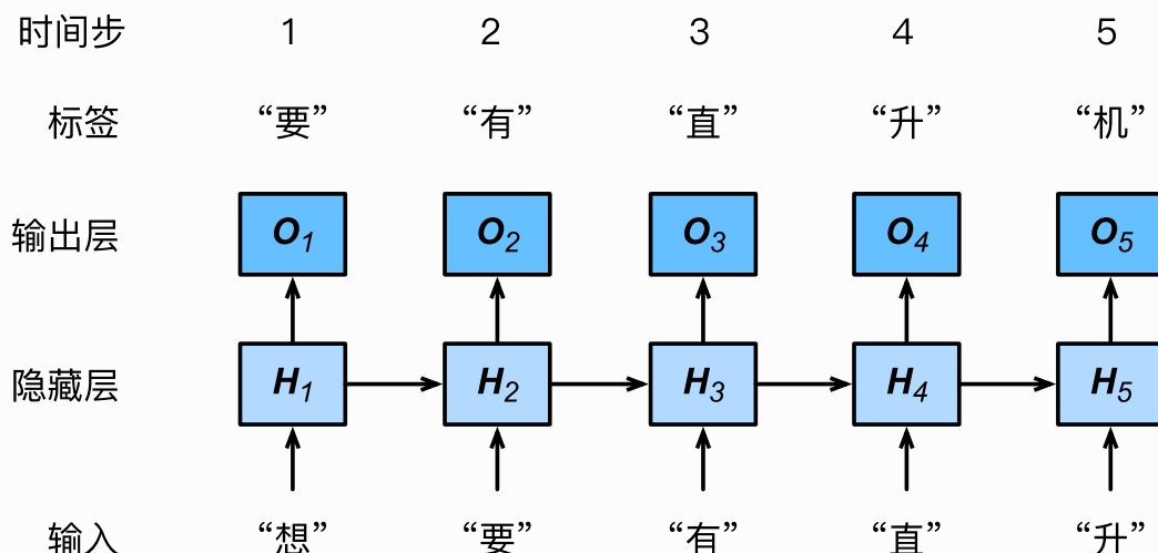
图6.2 基于字符级循环神经网络的语言模型。
