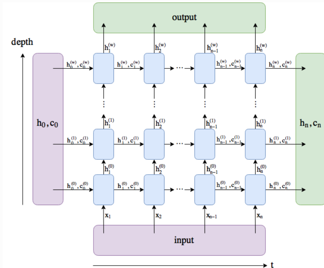
循环神经网络(以LSTM为例)的输出
