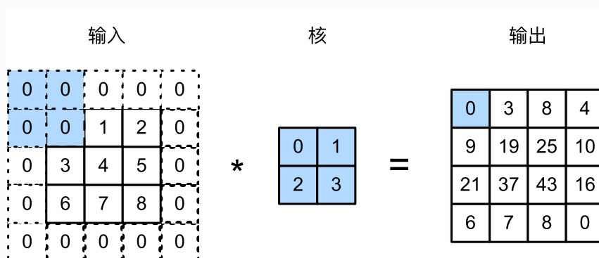
图5.2 在输入的高和宽两侧分别填充了0元素的二维互相关计算
