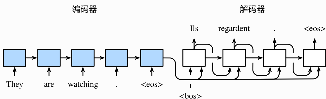
图10.8 使用编码器—解码器将句子由英语翻译成法语。编码器和解码器分别为循环神经网络接下来，我们分别介绍编码器和解码器的定义。
