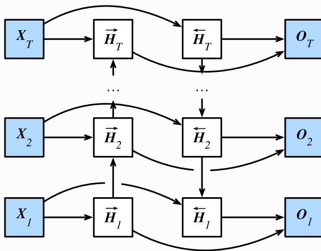
图6.12 双向循环神经网络的架构
