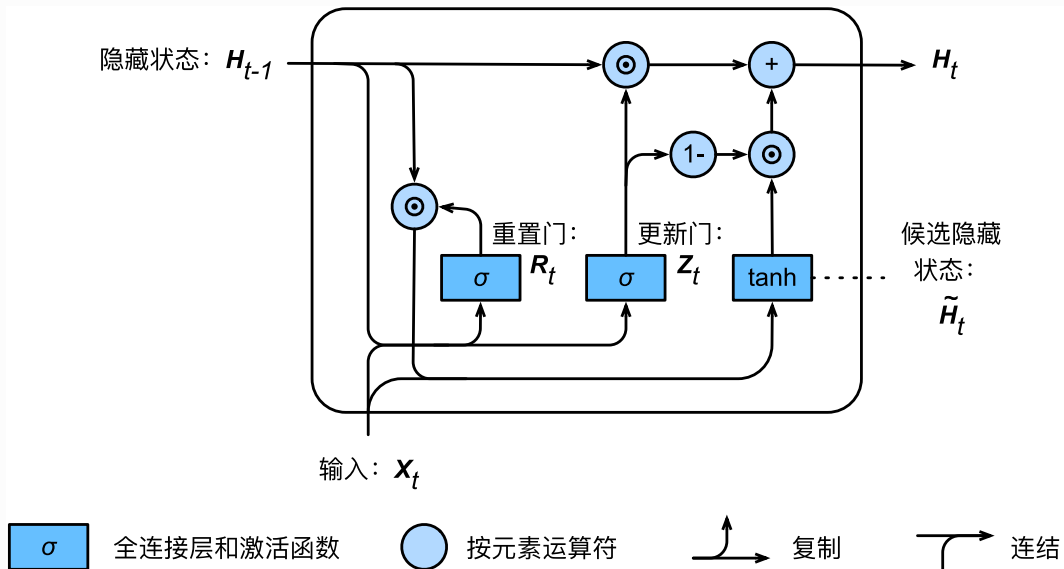
图6.6 门控循环单元中隐藏状态的计算
