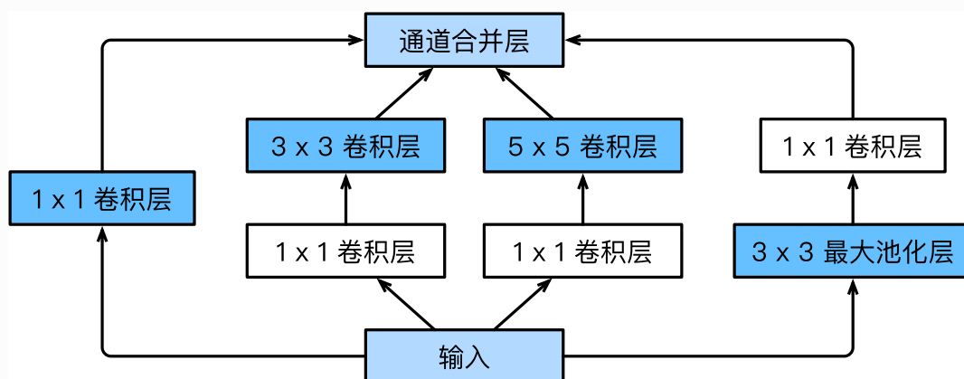
图5.8 Inception块的结构
