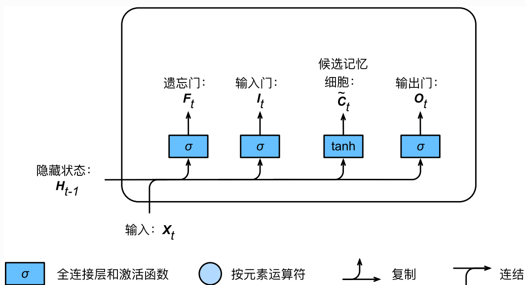
图6.8 长短期记忆中候选记忆细胞的计算
