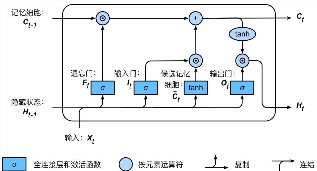
图6.10 长短期记忆中隐藏状态的计算
