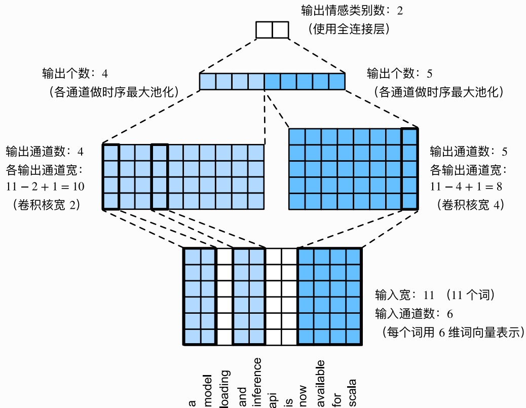
图10.7 textCNN的设计
