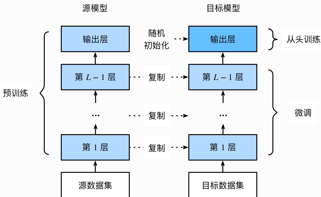
图9.1 微调
