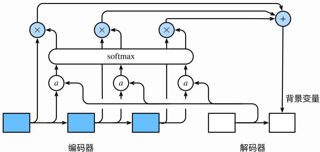
图10.12 编码器—解码器上的注意力机制
