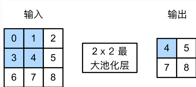
图5.6 池化窗口形状为 2 \times 2 的最大池化
