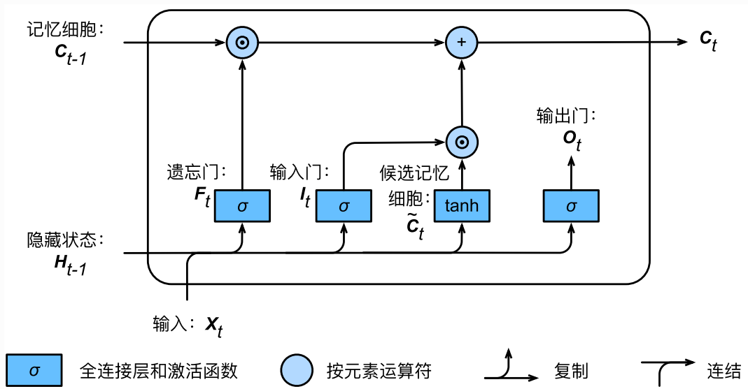
图6.9 长短期记忆中记忆细胞的计算
