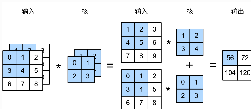
图5.4 含2个输入通道的互相关计算
