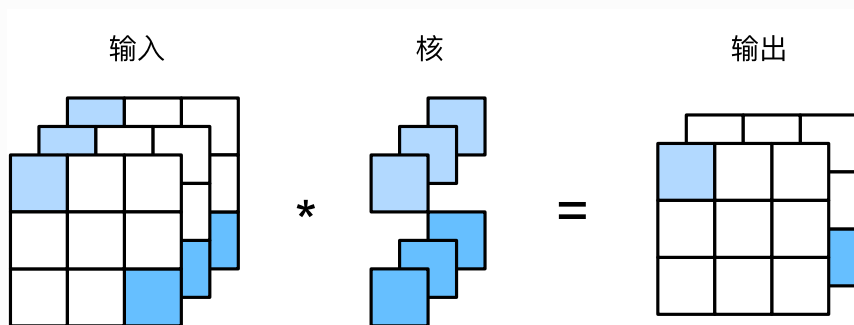
图5.5 1 \times 1 卷积核的互相关计算。输入和输出具有相同的高和宽
